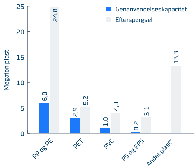
Figur 4: Efterspørgsel af plast generelt og genanvendelseskapacitet, opdelt efter polymerer. *Manglende data på kapacitet for resterende polymerer. (Plastics Recyclers Europe, 2023)
